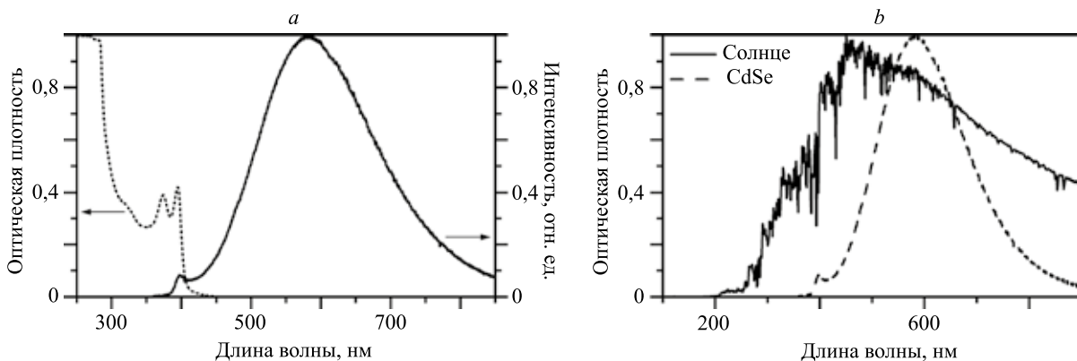
Рис. 1. Спектры поглощения (пунктирная кривая) и фотолюминесценции (сплошная кривая) наносвитков селенида кадмия (CdSe) ( a ); спектры излучения Солнца и фотолюминесценции исследуемых наносвитков CdSe ( b )
