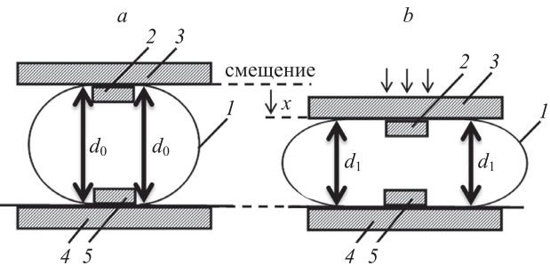
Рис. 2. Схема крепления оптоволокну ( a ) и его деформирования ( b ): 1 — оптическое волокно; 2, 3 — подвижные упоры; 4, 5 — неподвижные упоры
