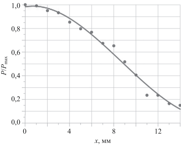
Рис. 6. Зависимость смещения x от относительной средней проходящей мощности P/P_{\max}
