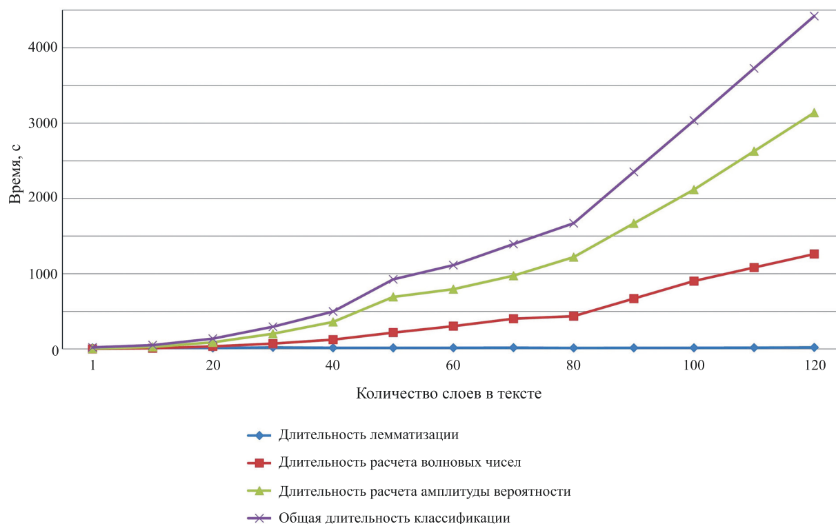
Рисунок. Длительность классификации в зависимости от длины текста Figure. Duration of classification depending on the text length
