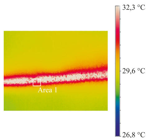
Рис. 8. Тепловое распределение на участке нижнего слоя, где Area 1 — выбранная область измерений Fig. 8. Thermal distribution in the area of the lower layer where Area 1 is the selected measurement area
