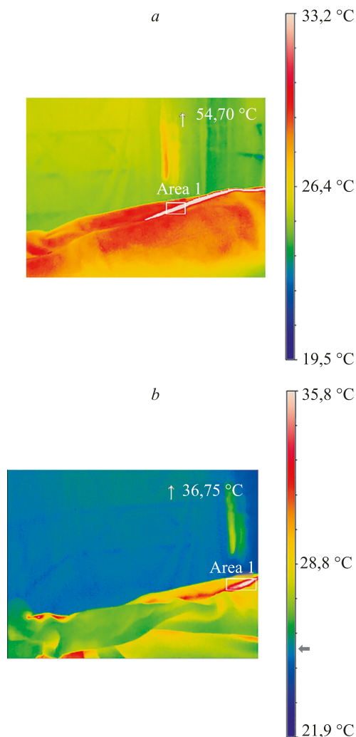
Рис. 9. Тепловое распределение на участках верхнего (a) и нижнего (b) слоев
