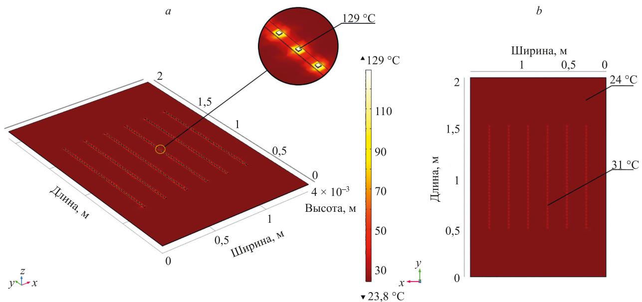
Рис. 5. Распределение температуры по поверхности объекта визуального отображения на верхнем (a) и нижнем (b) слоях. 129^\circ\text{C} и 31^\circ\text{C} — максимальные температуры в местоположении светодиода на верхнем и нижнем слоях; 4 \times 10^3 — координата по оси Z
