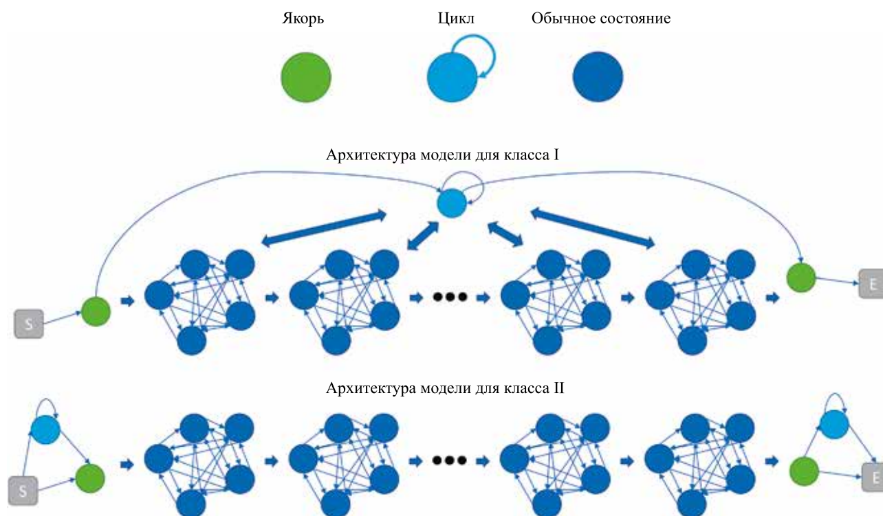
Рис. 5. Архитектура моделей
