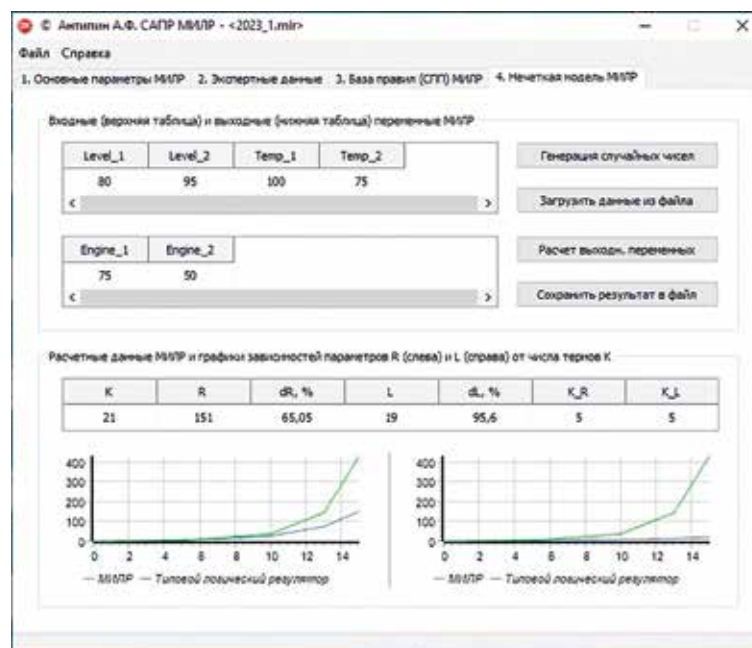
Рис. 7. Приложение для тестирования и симуляции работы многомерных интервально-логических регуляторов
