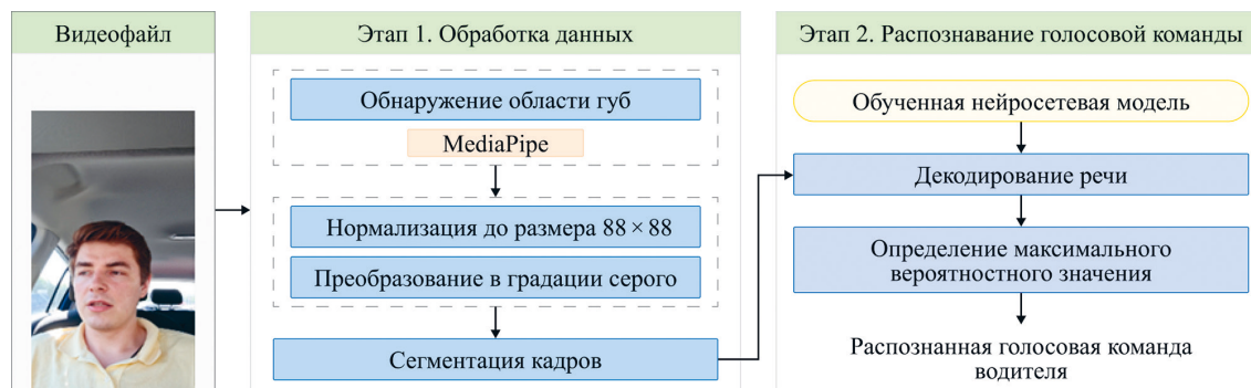
Рис. 1. Метод визуального распознавания команд водителя
