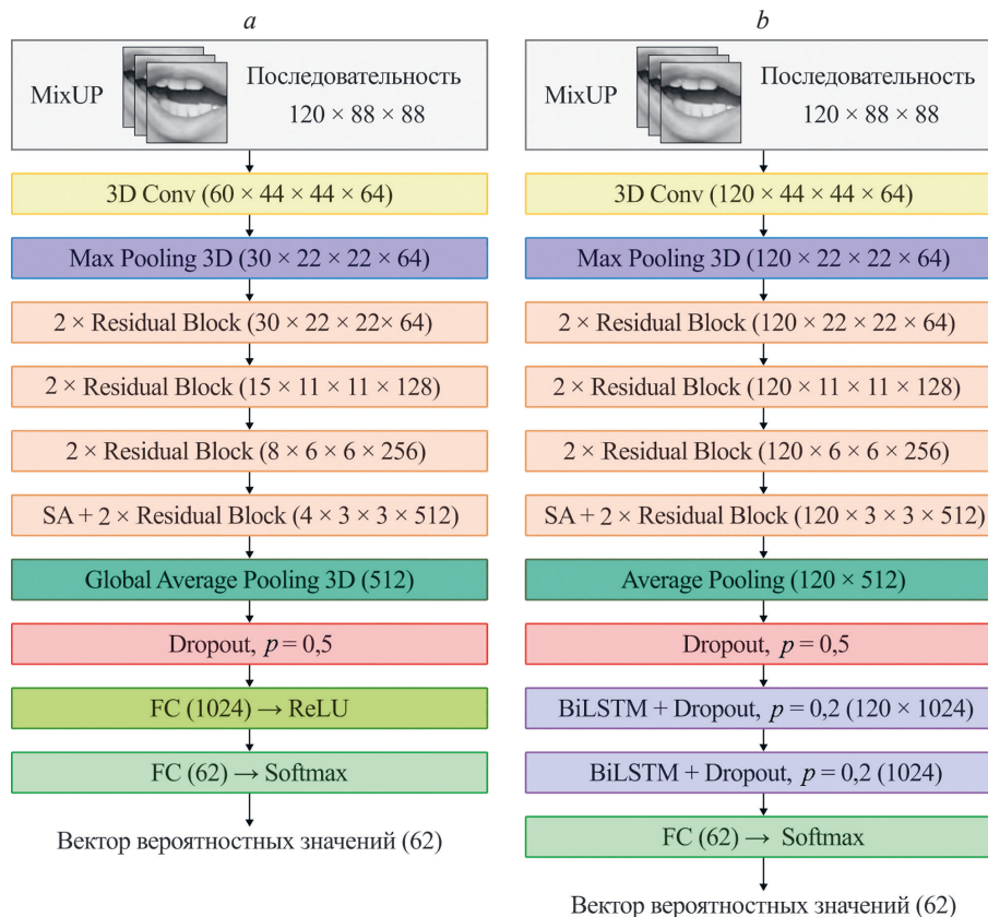
Рис. 2. Нейросетевые архитектуры: 3DResNet18 + SA (а); 3DResNet18 + SA+ BiLSTM (б)
