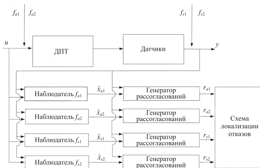
Рис. 2. Схема детектирования и локализации отказов
