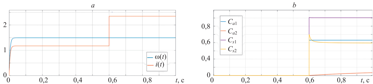
Рис. 7. Случай мультипликативного отказа датчика тока: выходные сигналы двигателя (а); коэффициенты направлений (b) Fig. 7. Case of current sensor multiplicative fault: motor output signals (a); direction coefficients (b)
