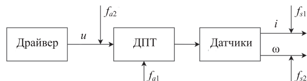
Рис. 1. Структурная схема модели исследуемого объекта
