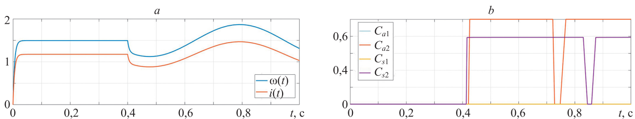
Рис. 5. Случай отказа при отклонении напряжения: выходные сигналы двигателя (а); коэффициенты направлений (б)
