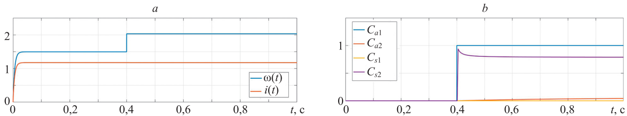
Рис. 4. Случай отказа по внешнему моменту сил: выходные сигналы двигателя (а); коэффициенты направлений (б)
