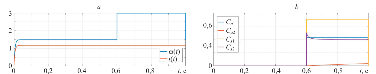
Рис. 6. Случай мультипликативного отказа датчика скорости: выходные сигналы двигателя (а); коэффициенты направлений (б)
