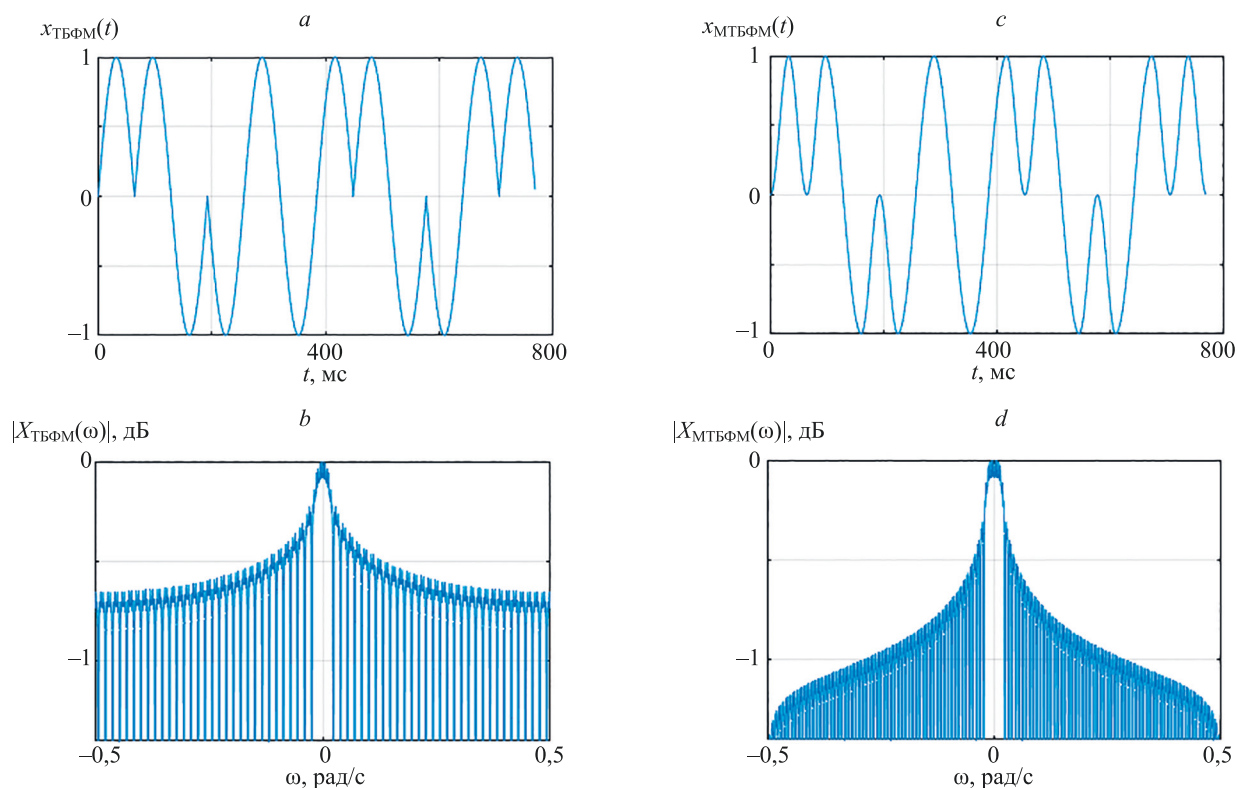
Рис. 7. Сравнение сигналов: трехпозиционной бинарной фазовой манипуляции x_{\text{TBPM}}(t) (а), модифицированной трехпозиционной бинарной фазовой манипуляции x_{\text{MTBPM}}(t) (с) и их нормированных по частоте модулей спектров |X_{\text{TBPM}}(\omega)| (b) и |X_{\text{MTBPM}}(\omega)| (d)
