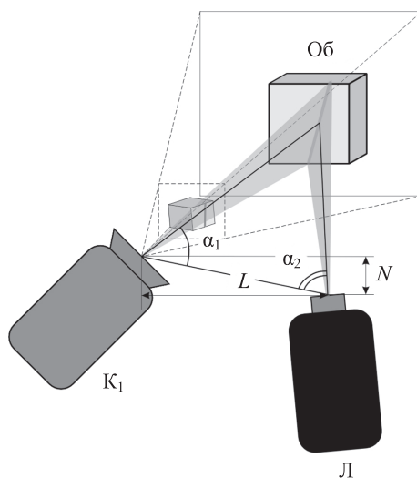
Рис. 2. Иллюстрация принципа лазерного сканирования.
