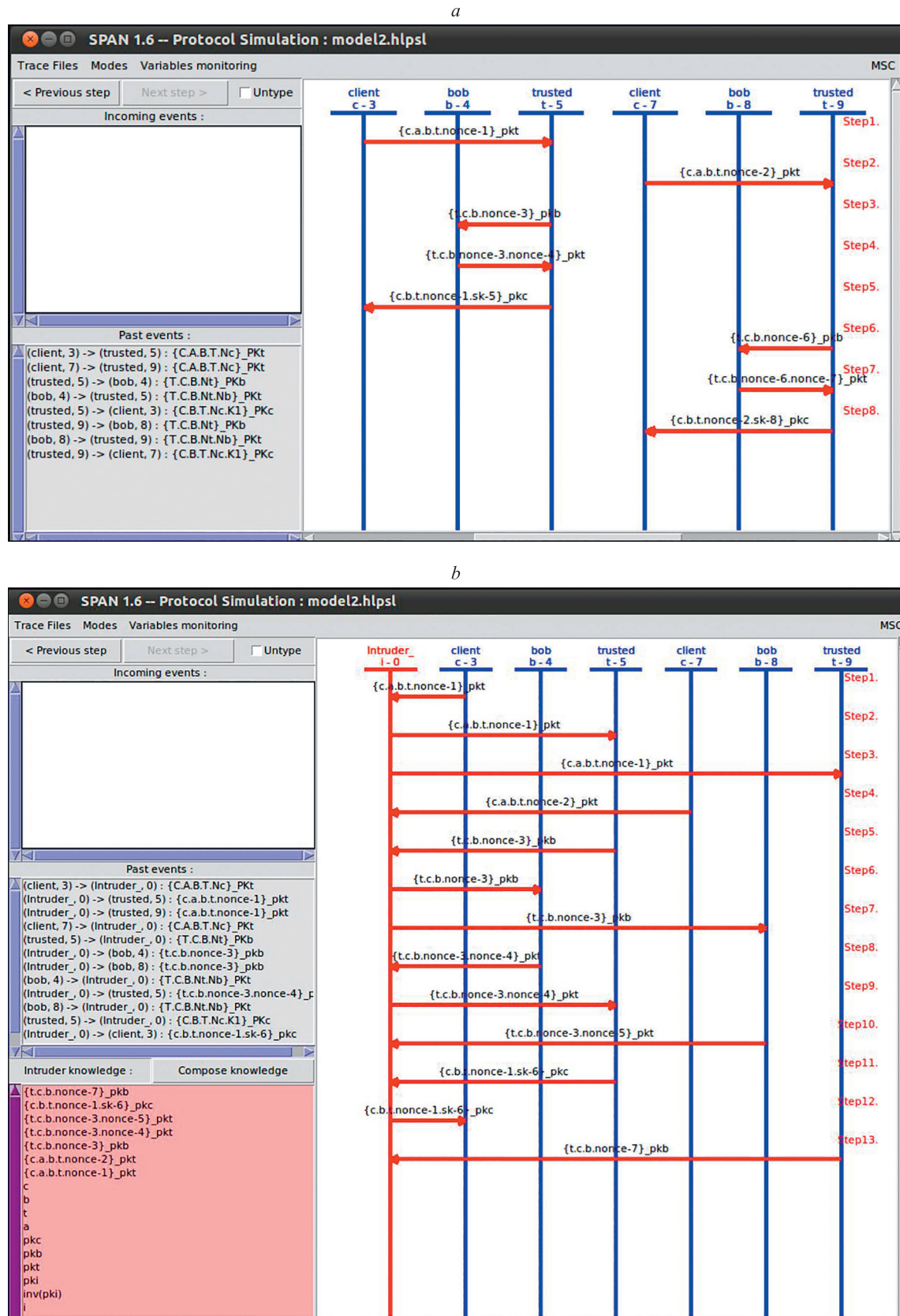
Рис. 6. Визуализация информационных потоков взаимодействия сценария 2 в среде AVISPA: без нарушителя информационной безопасности (а); с нарушителем информационной безопасности (b)
