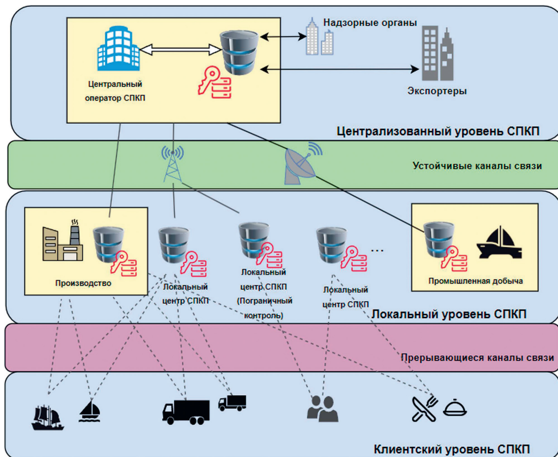
Рис. 1. Обобщенная архитектура системы прослеживаемости качества продукции
