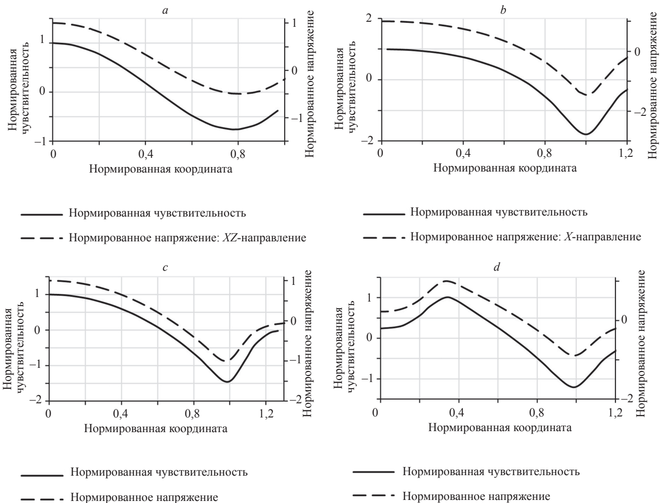
Рис. 3. Графики чувствительности для мембран: квадратной формы ( XZ -направление) (а); квадратной формы ( X -направление) (б); круглой (с); круглой с жестким центром (д)
